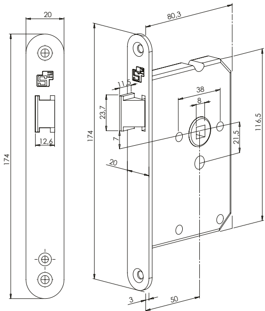
Loopslot
