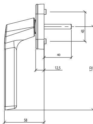
Raamgreep
