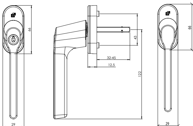
Zelfstellende raamgreep
