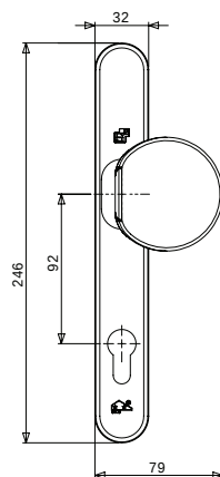
Buitenzijde
