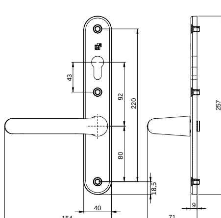
Binnenzijde
