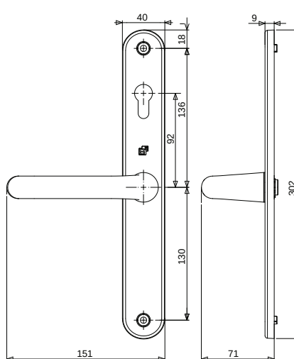
Binnenzijde
