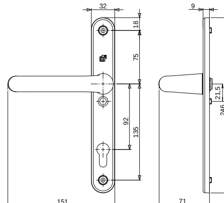
Binnenzijde
