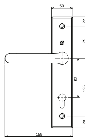
Binnenzijde
