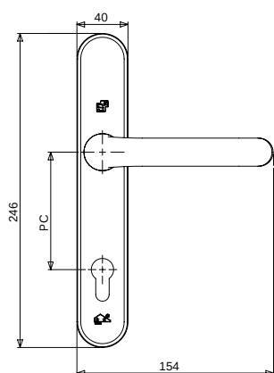
Buitenzijde
