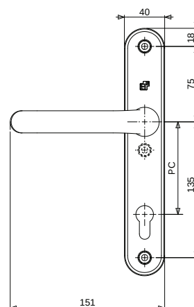
Binnenzijde
