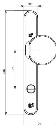
Buitenzijde
