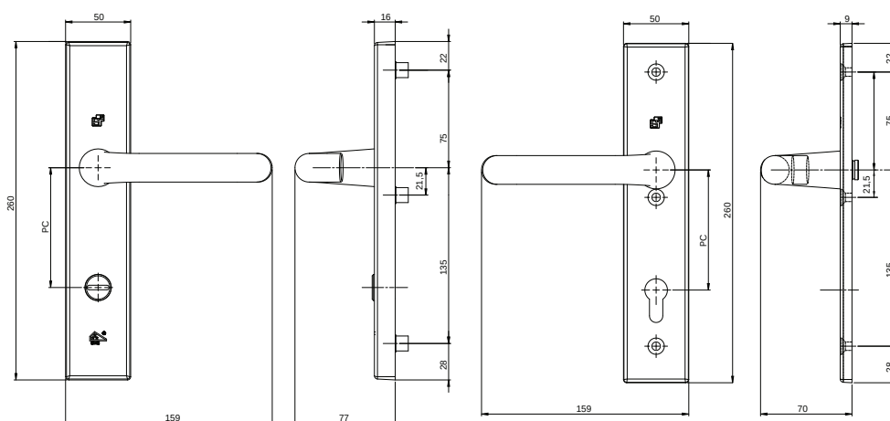
Buitenzijde
