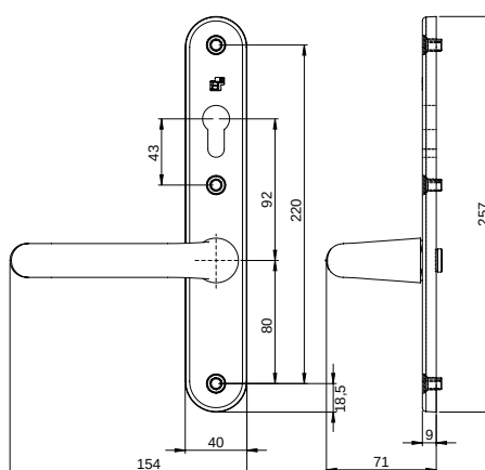
Binnenzijde
