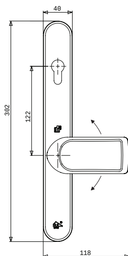
Buitenzijde
