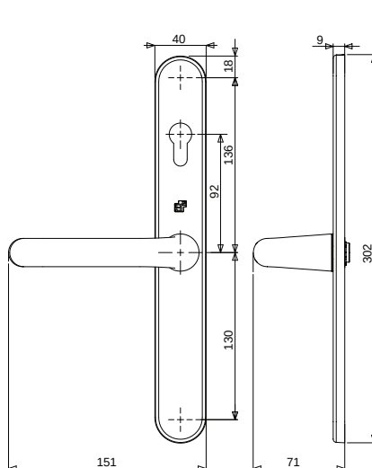
Binnenzijde
