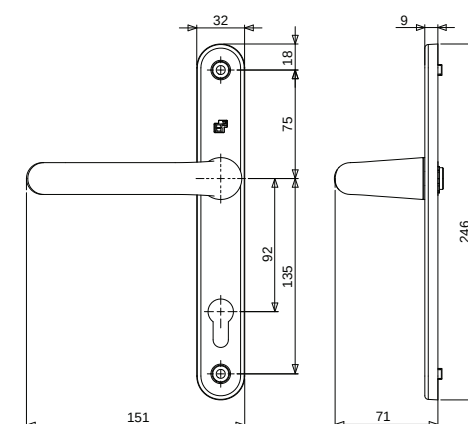
Binnenzijde
