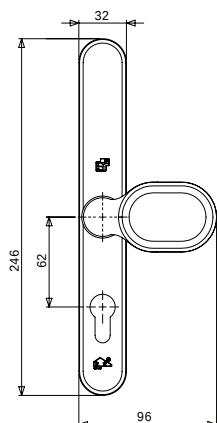
Buitenzijde
