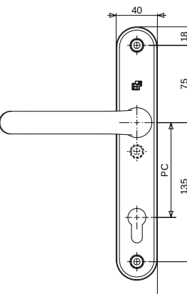
Binnenzijde
