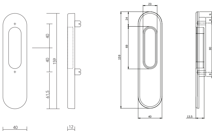
Opbouwkom
