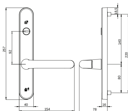
Buitenzijde
