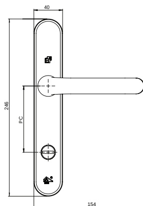
Buitenzijde
