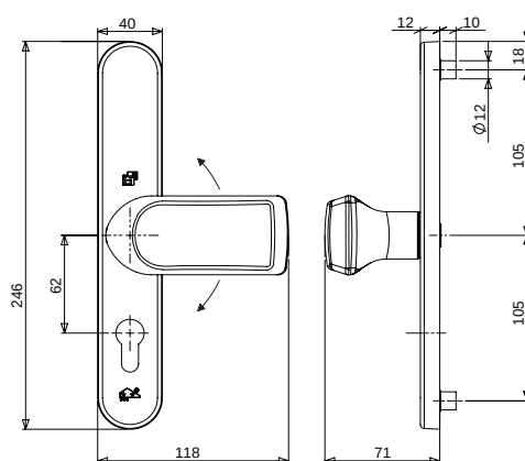
Buitenzijde
